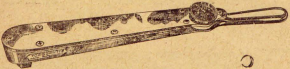
Torquímetros para porcas e parafusos com escalas em libras-pés e metro-Kg, com lâmpadas de regulagem; de 15 libras" a 2.000 libras-pés.
