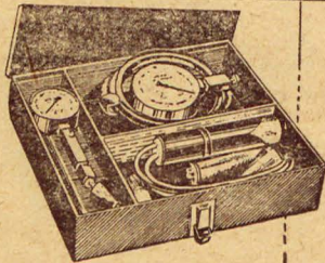
Analísadores para medir compressão, vácuo, bomba de gasolina e lâmpada Neon
